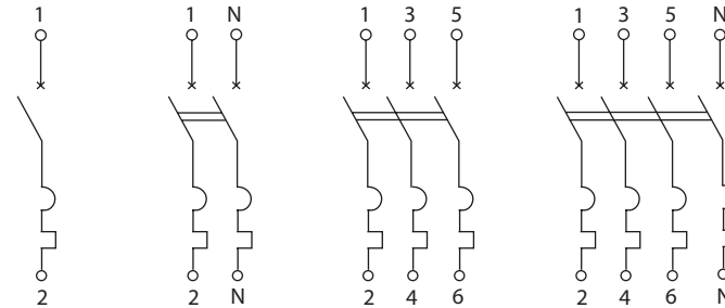
Рис. 3 - 1 полюс
