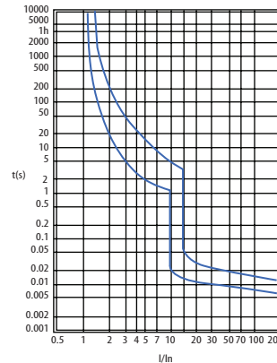
Рис. 2 - Характеристика D
