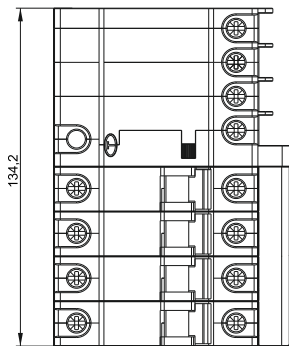
а) АД14 50-63 А
