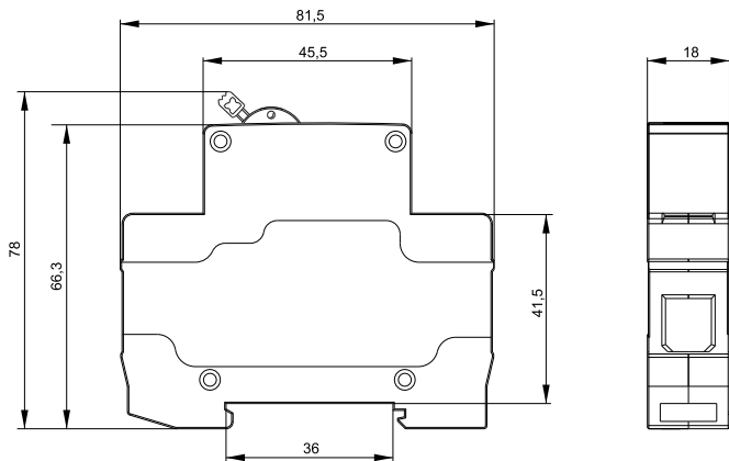
Рисунок 1 – Габаритные и установочные размеры выключателя
