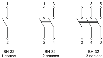
Рисунок 2 – Схема электрическая выключателя
