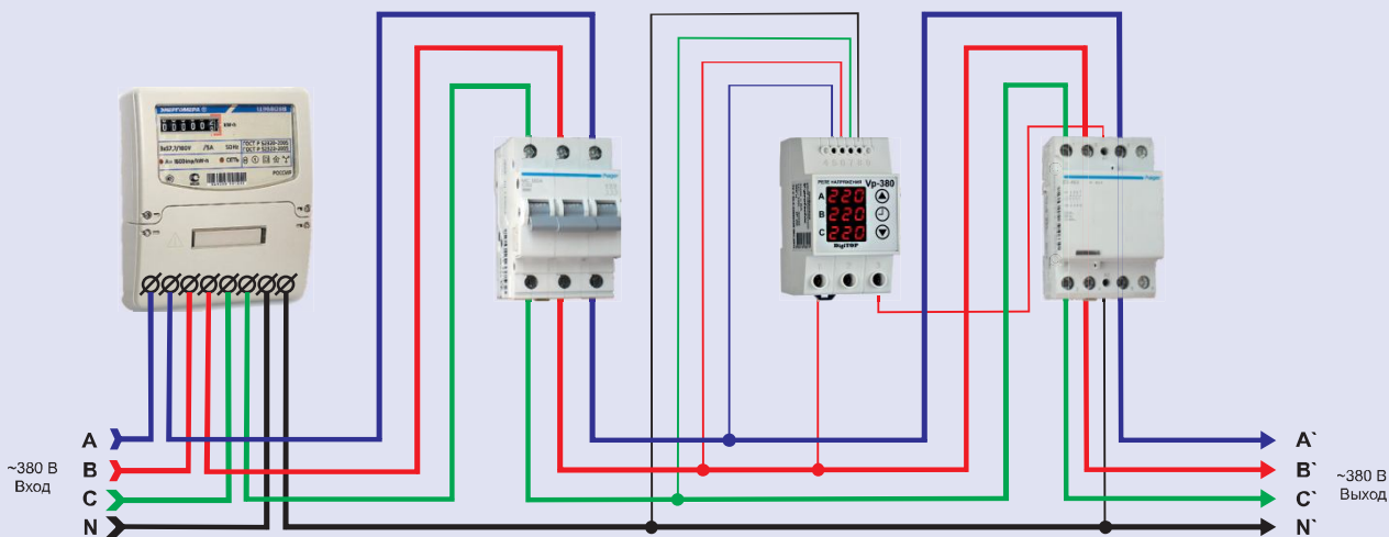
Защита 3-фазных потребителей
