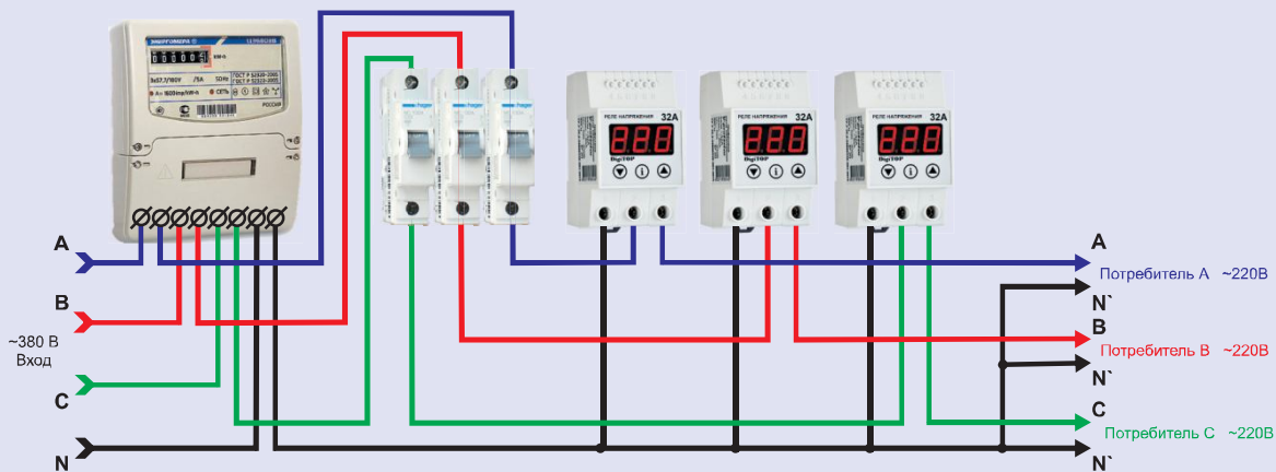
Защита 3-фазной сети с 1-фазными потребителями
