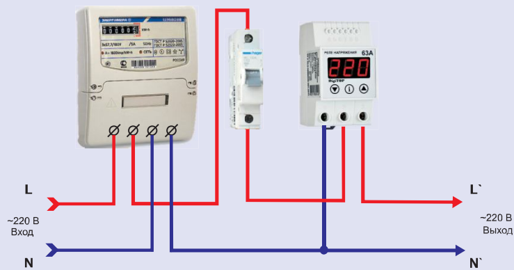
Защита 1-фазной сети
