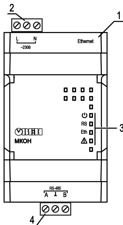
Рисунок 7.1 – Общий вид шлюза
