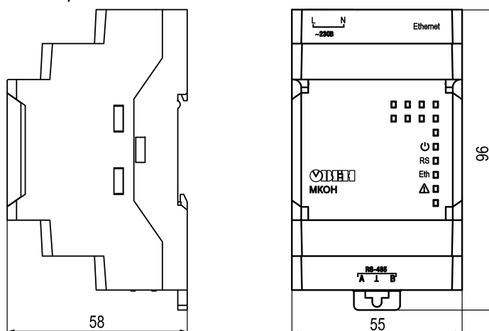
Рисунок 5.1 – Габаритные размеры
