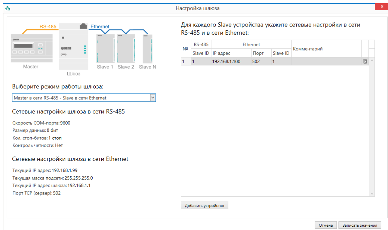
Рисунок 8.12 – Настройки шлюза Master RS-485 - Slave Ethernet
