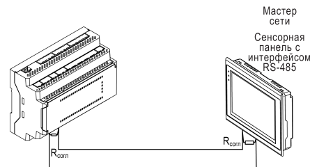
Рисунок 5 – Типовая схема подключения в режиме Slave
