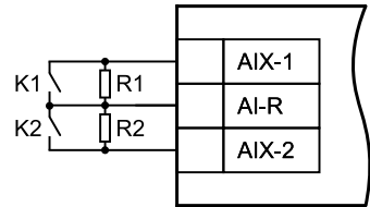
Рисунок 7 – Подключение «сухих контактов»
