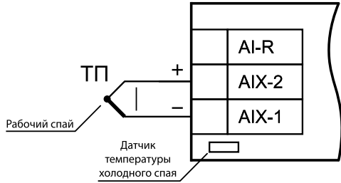
Рисунок 3 – Схема подключения термоэлектрического преобразователя
