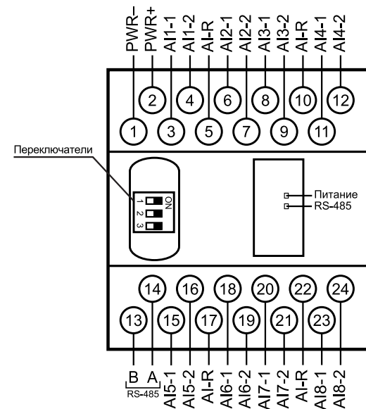
Рисунок 1 – Назначение контактов клеммника
