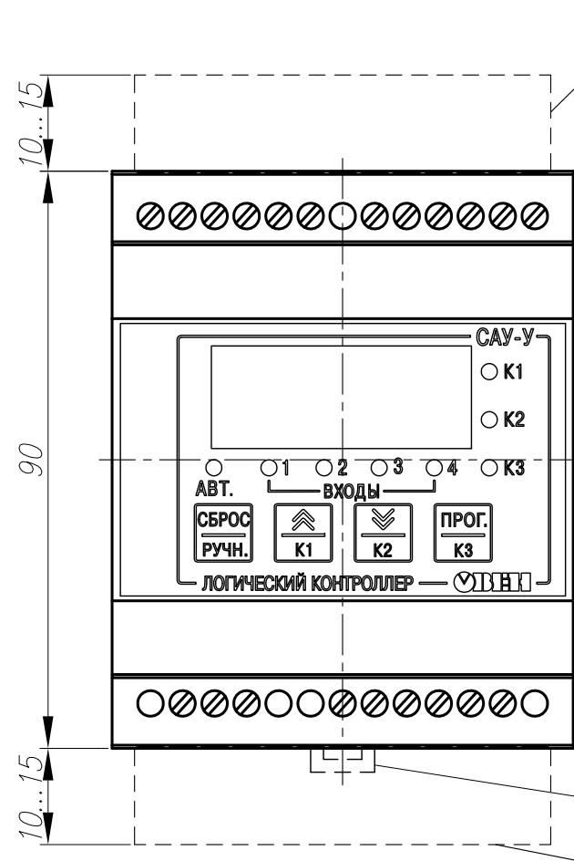
Вид спереди
