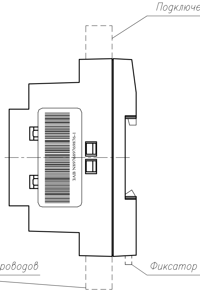
Вид справа
