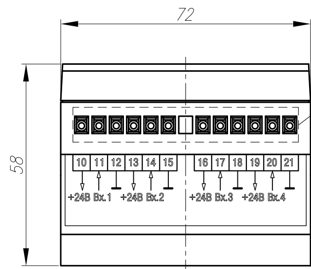
Вид сверху
