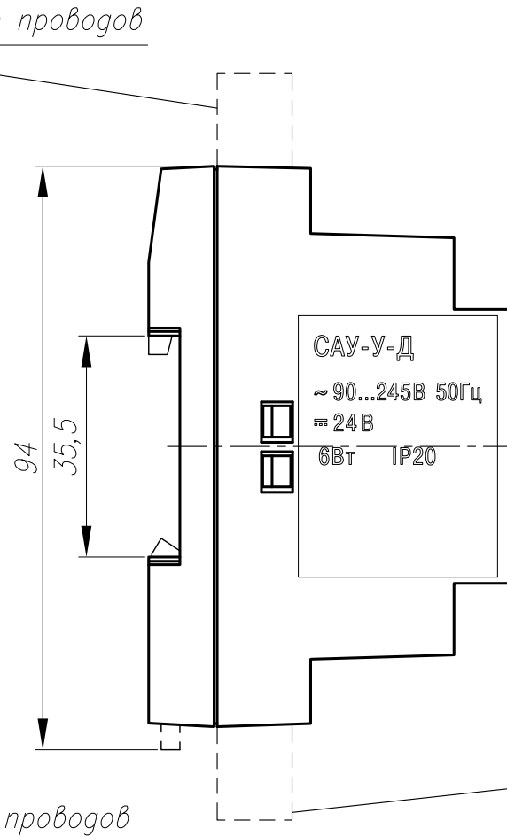
Вид слева
