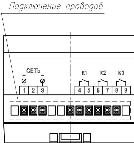
Вид снизу
