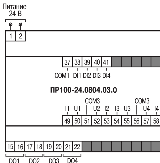
Рисунок А.1 – Расположение контактов для ПР100-24.0804.03.0
