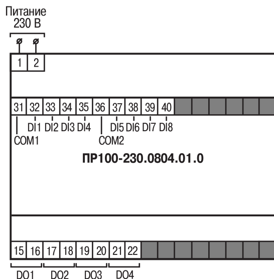
Рисунок А.5 – Расположение контактов для PR100-230.0804.01.0
