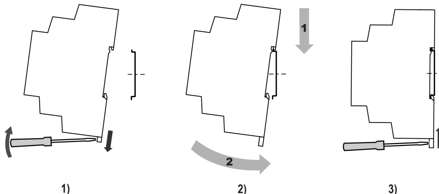
Рисунок 5.2 – Установка прибора
