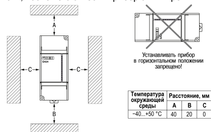
Рисунок 4.1 – Рекомендации по размещению прибора
