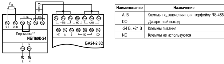
Рисунок 5.1 – Схема подключения
