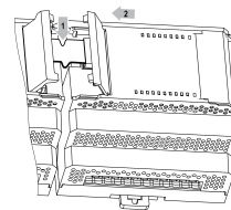
Рисунок 5 – Укладка шлейфа в углубление
