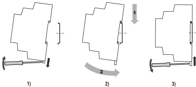
Рисунок 1 – Установка прибора
