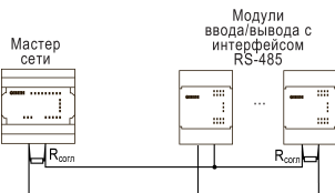
Рисунок 10 – Типовая схема подключения для PR100 в режиме Master
