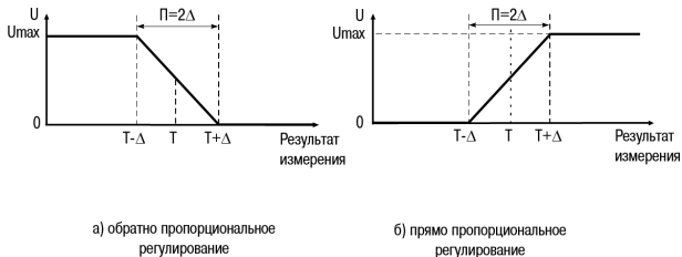
Рисунок 7.9 – Принцип формирования выходного сигнала П-регулятора для приборов с ВУ типа У
