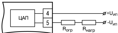
Рисунок 5.5 – Схема подключения ВУ типа И
