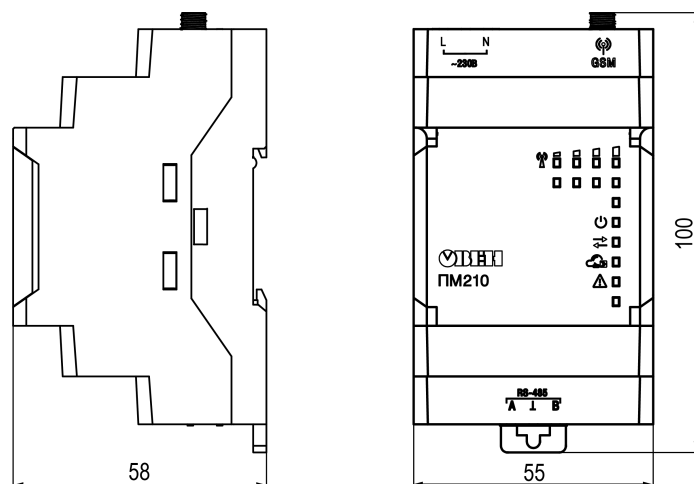
Рисунок 4.1 – Габаритные размеры
