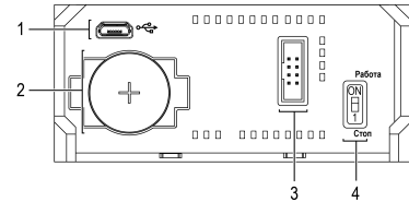
Рисунок 10 – Лицевая панель под крышкой
