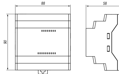
Рисунок 2 – Габаритные размеры
