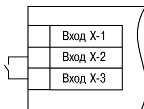
Рисунок 5.10 – Схема подключения к дискретному входу
