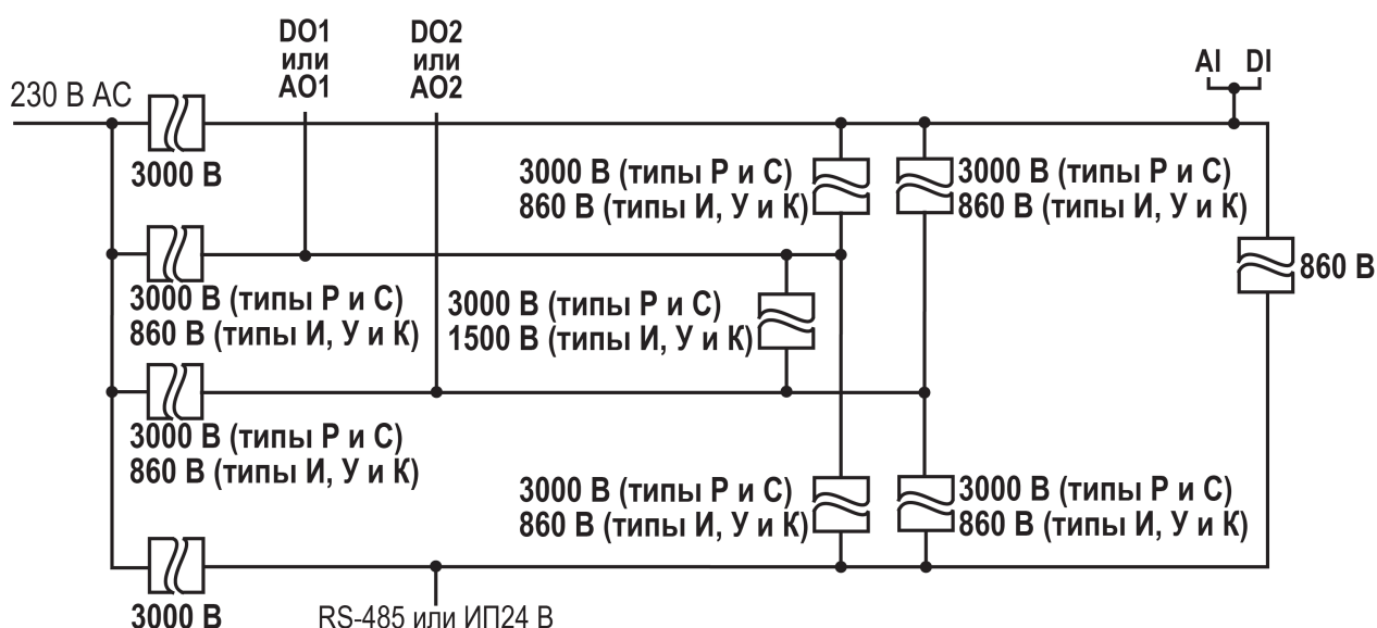
Рисунок 5.3 – Схема гальванической развязки (выходы кроме типа «Т»)
