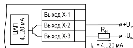
Рисунок 5.23 – Подключение к ВУ типа «И»
