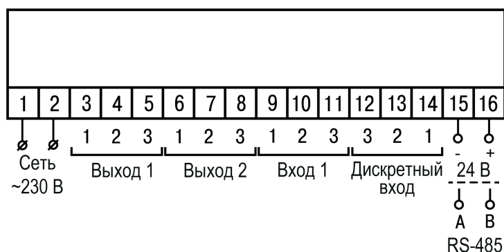
Рисунок 5.4 – Общая схема подключения ТРМ10–Щ1/Щ2
