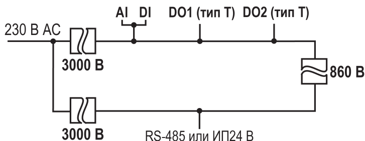
Рисунок 5.2 – Схема гальванической развязки (выход типа «Т»)
