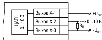
Рисунок 5.25 – Схема подключения нагрузки к ВУ типа «У»
