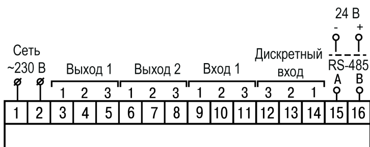
Рисунок 5.7 – Общая схема подключения ТРМ10–Н
