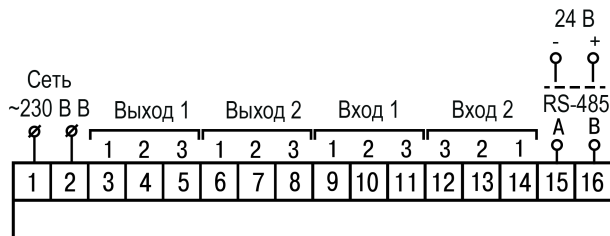
Рисунок 5.7 – Общая схема подключения ТРМ12–Н
