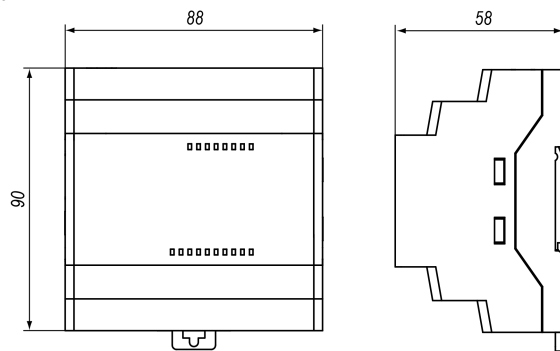
Рисунок 3 – Габаритные размеры
