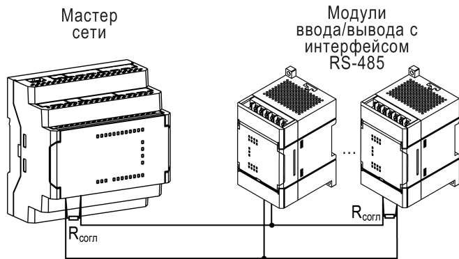
Рисунок 9 – Типовая схема подключения для ПР100 в режиме Master
