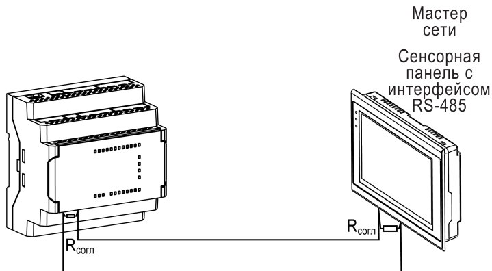
Рисунок 8 – Типовая схема подключения для ПР100 в режиме Slave
