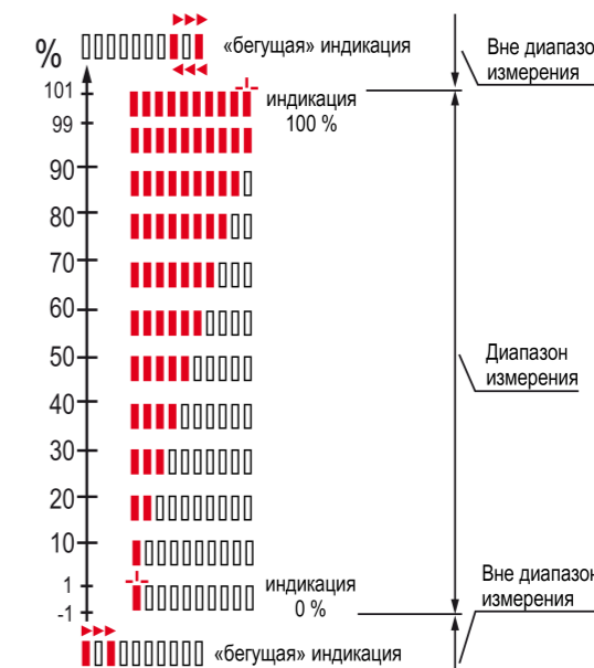
Рисунок 8.1 – Отображение измеряемого сигнала
