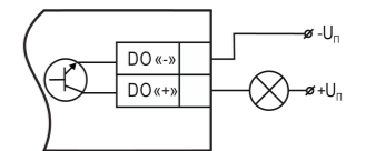
Рисунок 5.6 – Схема подключения выходного устройства
