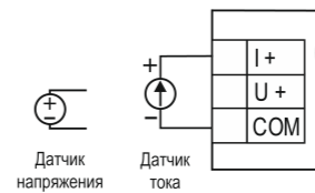
Рисунок 5.5 – Схемы подключения входных сигналов
