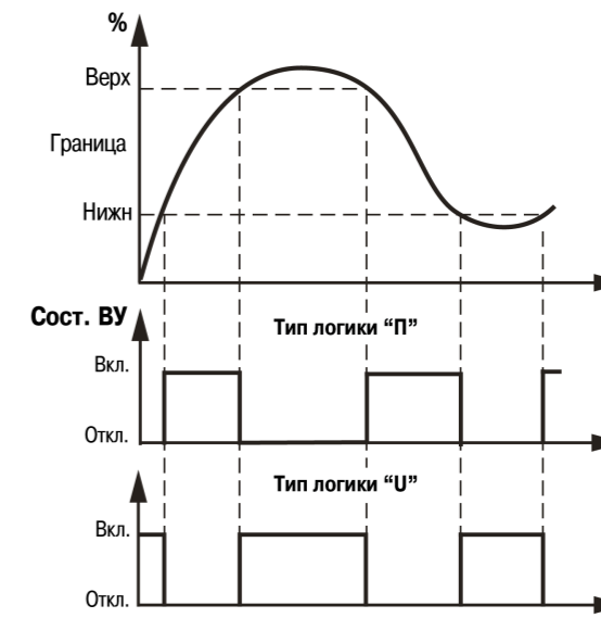
Рисунок 7.6 – Типы логики работы ВУ
