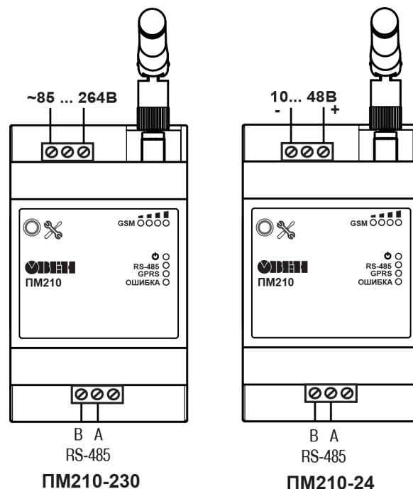
Рисунок 5.1 – Назначение клемм
