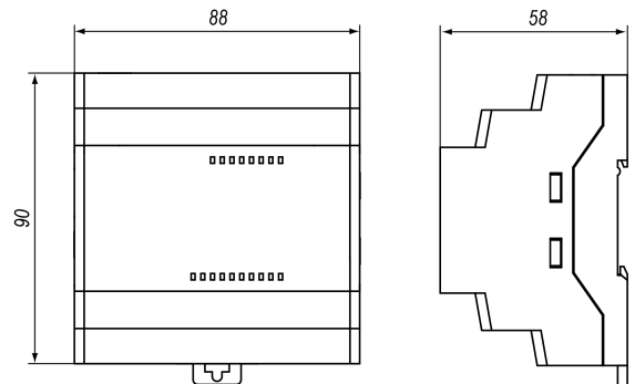
Рисунок 3 – Габаритные размеры
