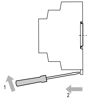
Рисунок 2 – Демонтаж прибора
