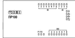
Рисунок 10 – Лицевая панель прибора
