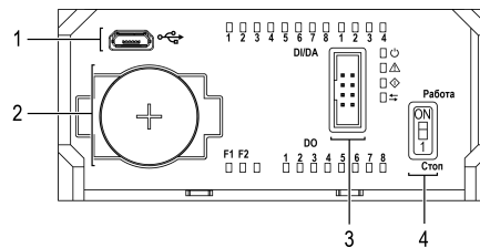
Рисунок 9 – Лицевая панель под крышкой
