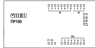
Рисунок 12 – Лицевая панель прибора
