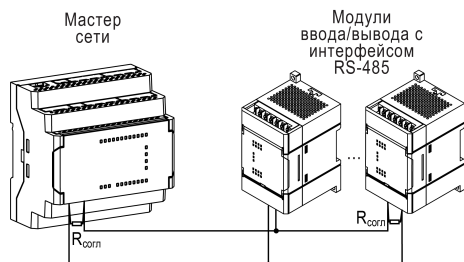
Рисунок 11 – Типовая схема подключения для PR100 в режиме Master
