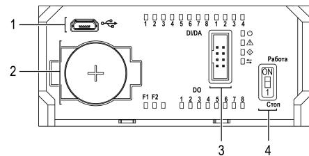
Рисунок 13 – Лицевая панель под крышкой
