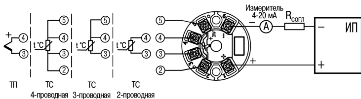
Рисунок 6.3 – Подключение прибора
