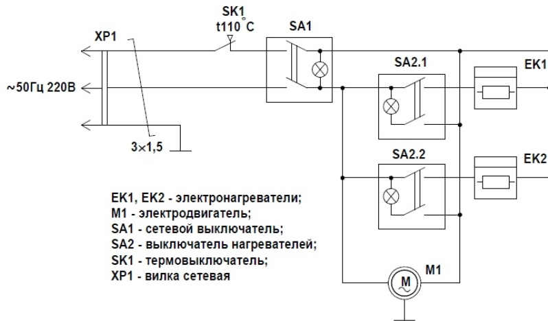
Рис. 1 Схема электрическая
