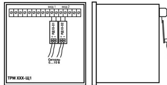
Рисунок 3.2 – Подключение делителей к двухканальному ТРМ в корпусе Щ1
