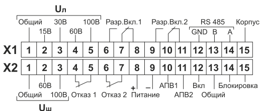
Рис. 2 Схема подключения устройства «Орион-КС»
