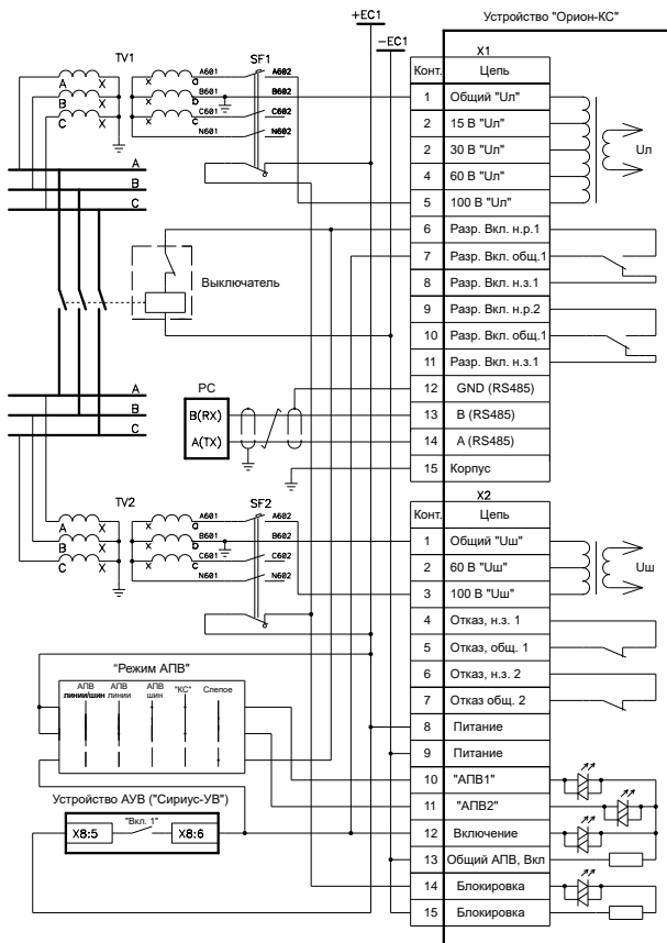
Рисунок 3. Схема подключения устройства «Орион-КС» при контроле синхронизма между линией и шиной, или между двумя секциями шин (с установкой контактов выходного реле «Разреш. Вкл.» непосредственно в цепь включения выключателя)
