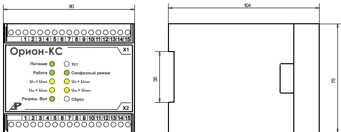
Рис. 1 Внешний вид и габаритные размеры устройства «Орион-КС»
