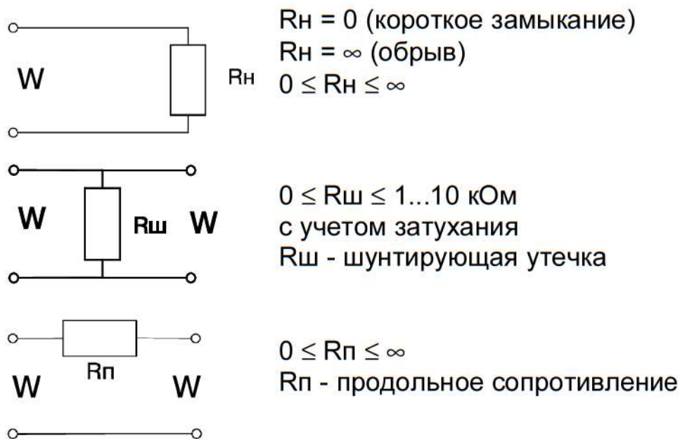
Рисунок 3 - Эквивалентные схемы повреждений
