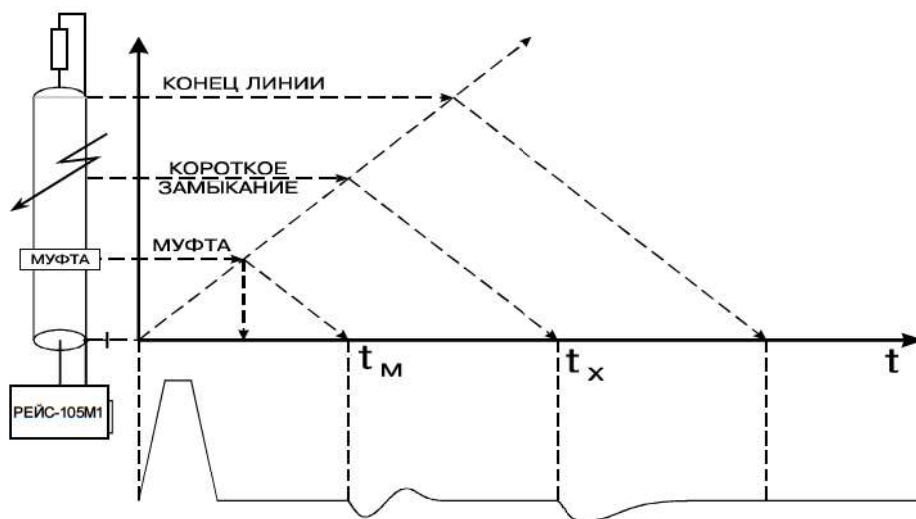
Рисунок 2 - Рефлектометрический метод определения места повреждения
