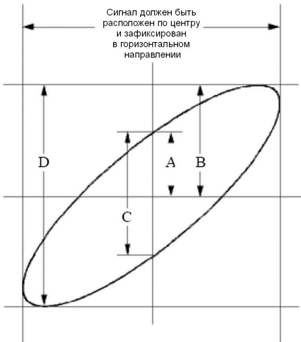
Рисунок 7.6. Фигура Лиссажу
