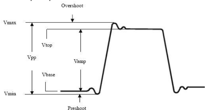
Рисунок 5.68. Параметры напряжения
