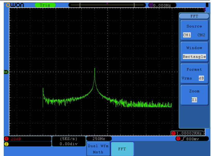
Рисунок 5.10. Быстрое преобразование Фурье с прямоугольным окном
