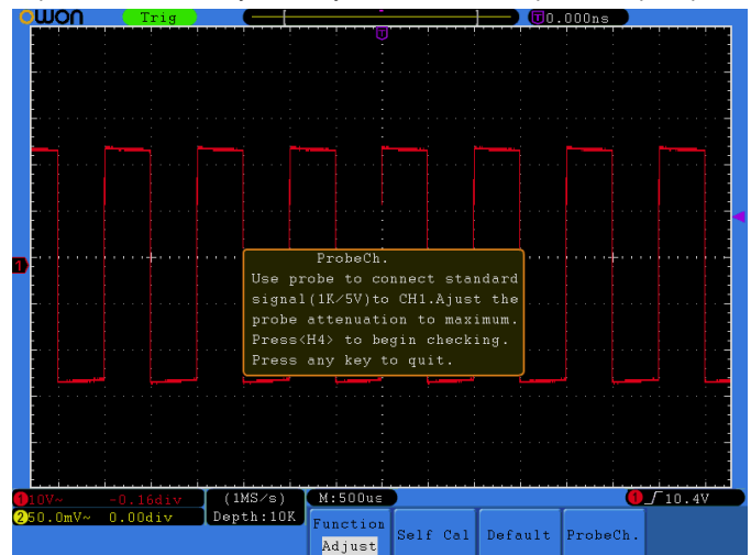
Рисунок 5.60. Проверка щупа.
