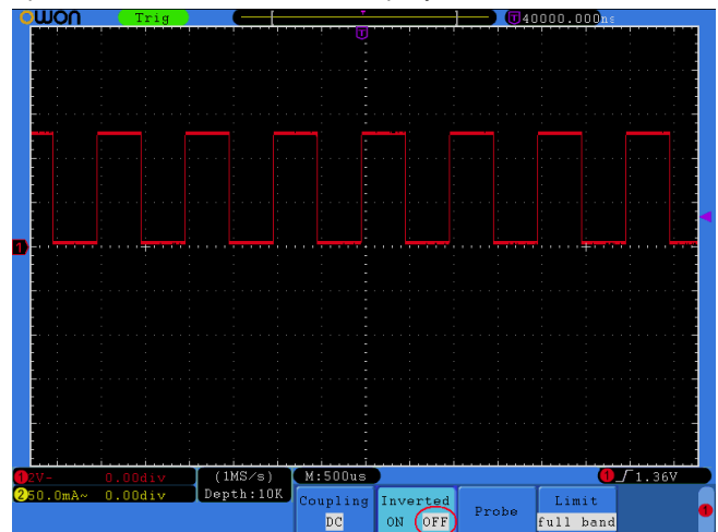
Рисунок 5.6. Нормальная осциллограмма
