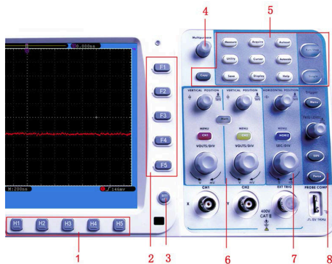
Рисунок 4.5. Панель управления
