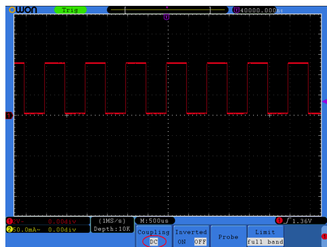
Рисунок 5.2. Вид осциллограммы в режиме связи по постоянному току
