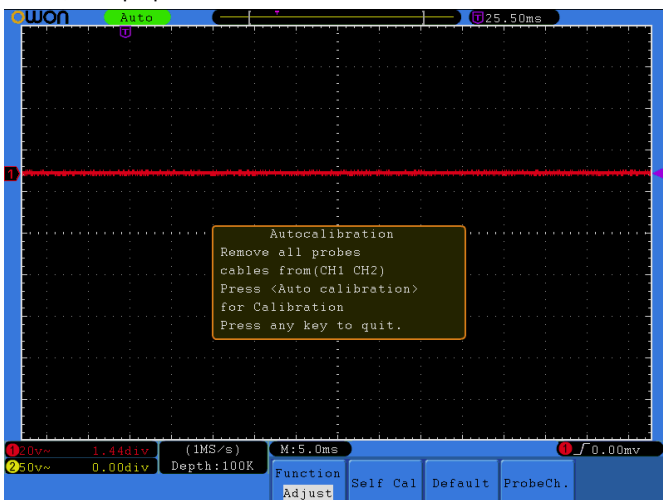
Рисунок 5.59. Автокалибровка осциллографа.
