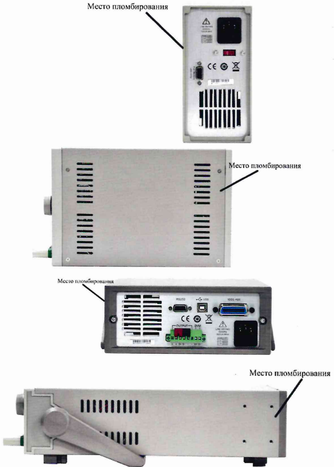
Рисунок 2 – Схема пломбировки источников от несанкционированного доступа
