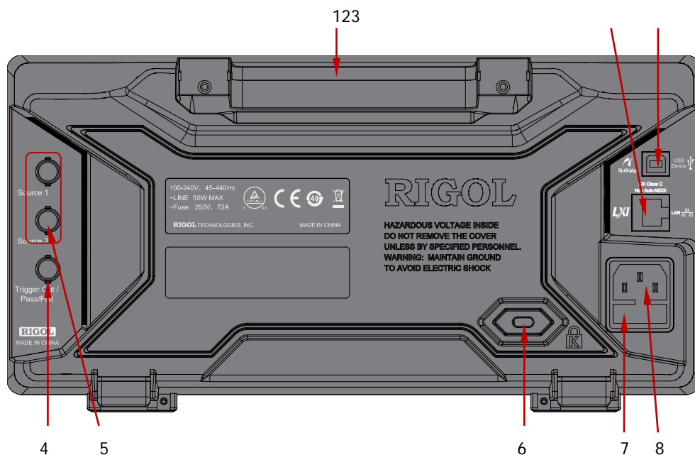
Рис. 0-100 Общий обзор задней панели.
