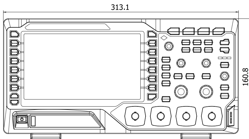
Рис. 0-1 Вид спереди
