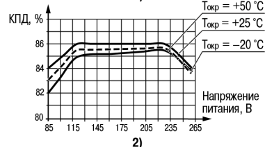
Рисунок 7 - График зависимости КПД от напряжения питания и температуры окружающей среды: (1) БП60А-12, (2) БП60А-24
