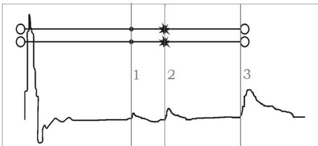
Рисунок 6-1 Муфты, скрутки, обрыв
