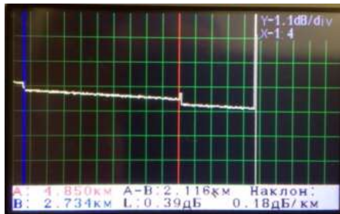
Рис. 14 Измерение длины и затухания участка линии
