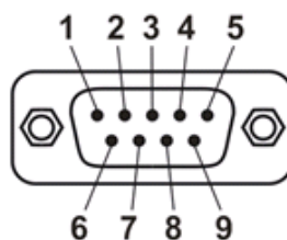
Рисунок 3.6 Разъем подключения к компьютеру по RS-232
