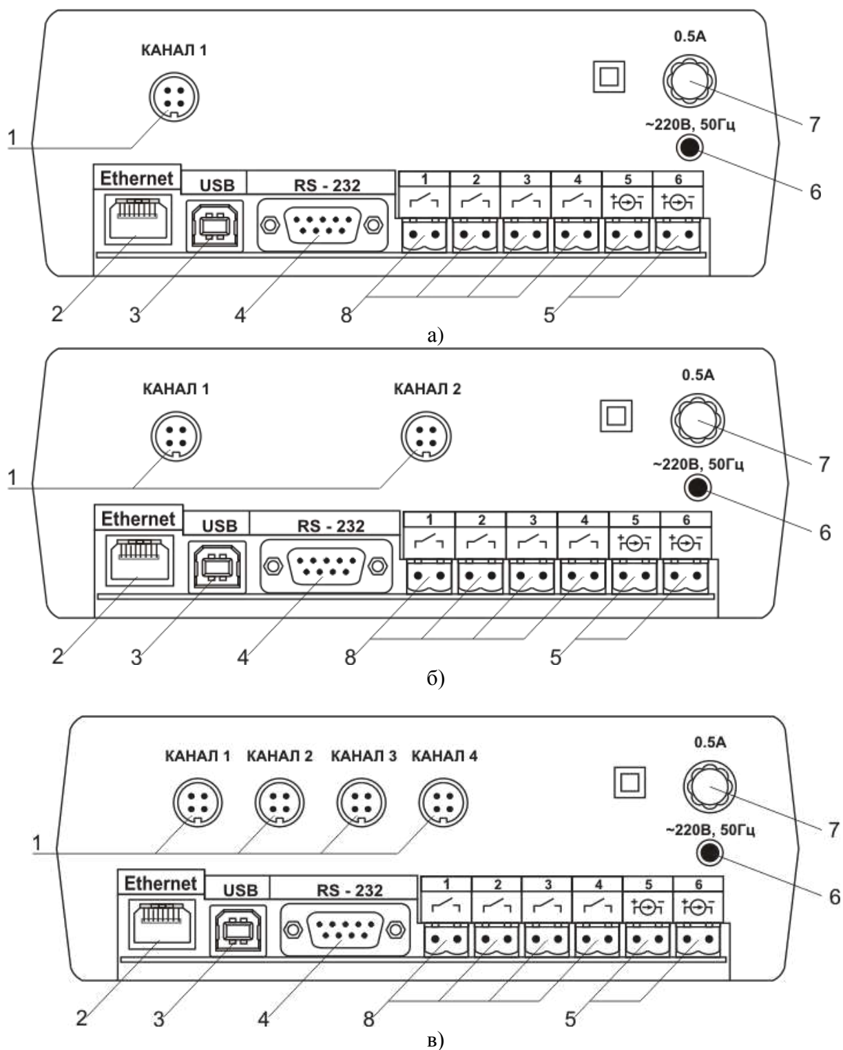
Рисунок 3.4 Вид задних панелей газоанализаторов ПКГ-4 /Х-Т-К-4Р-2А-Е (3):
