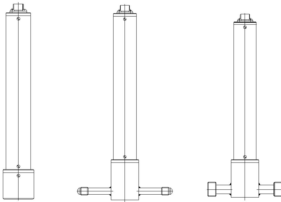
Рисунок 3.16 Измерительные преобразователи концентрации ИПК-03, ИПК-04-М8, ИПК-04-М16 (по порядку слева направо)
