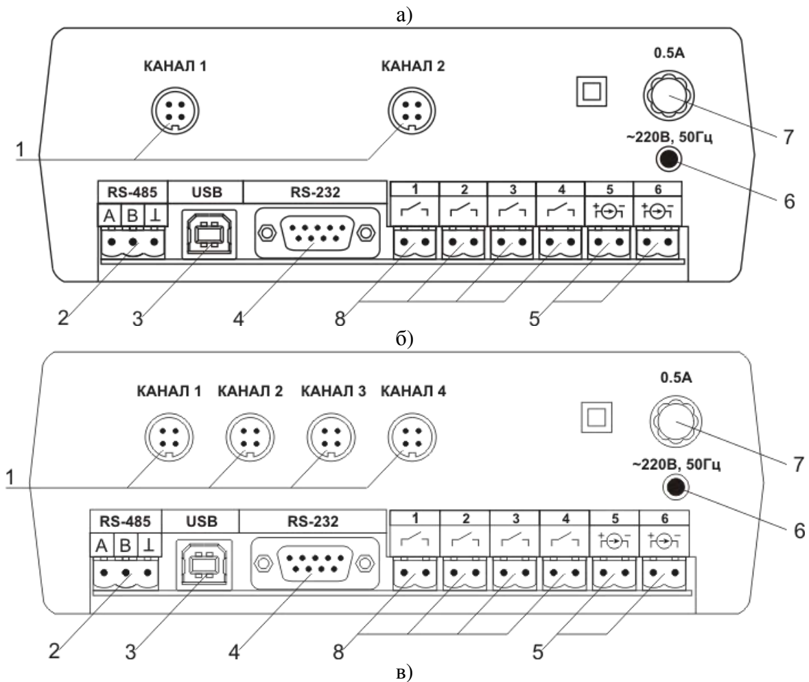
Рисунок 3.3 Вид задних панелей газоанализаторов ПКГ-4 /X-T-K-4P-2A (3):
