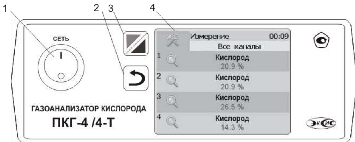
Рисунок 3.1 Вид лицевой панели газоанализатора:
