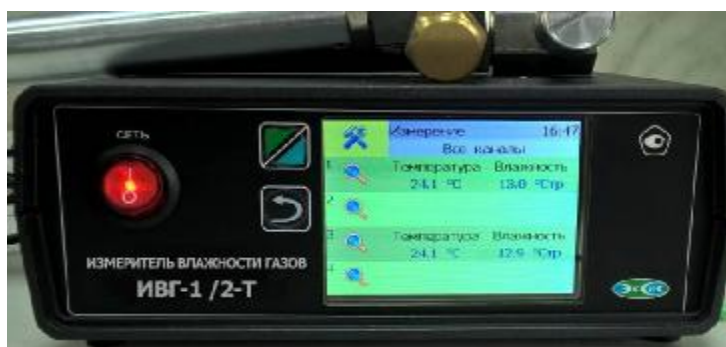
Рисунок 13 - Общий вид модификация ИВГ-1 /X исполнение ИВГ-1 /2-T
