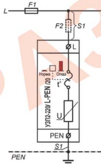
Рис.2 Схема подключения для однофазной сети
