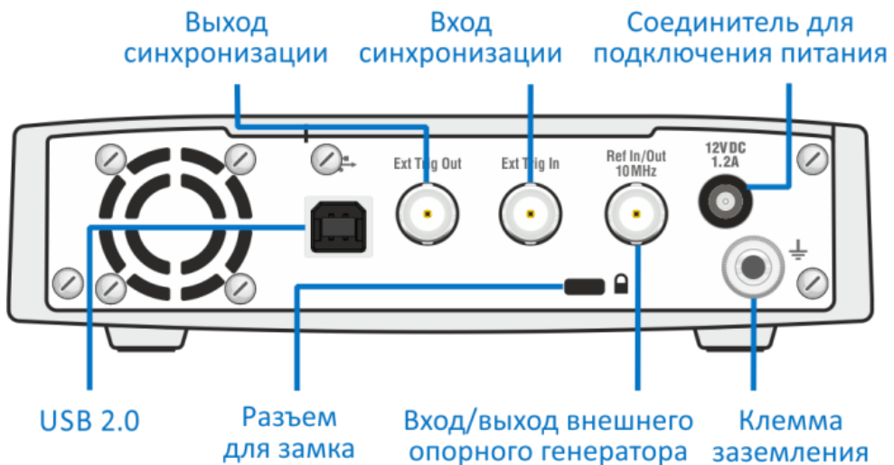
Рисунок 4.2 Задняя панель
