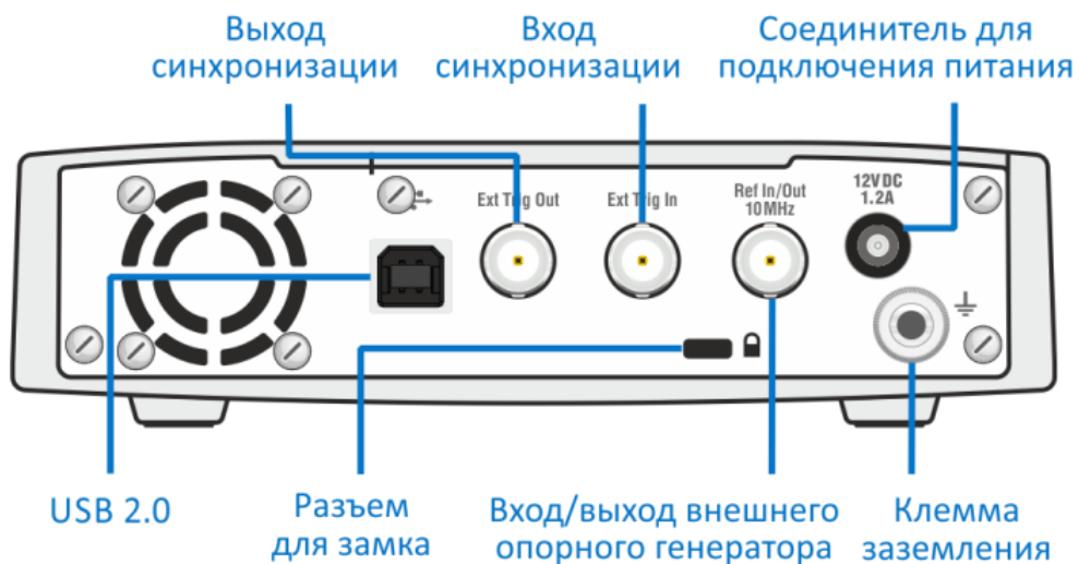
Рисунок 4.6 Задняя панель
