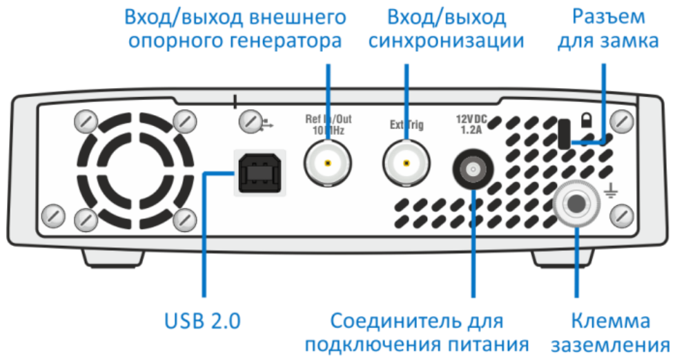
Рисунок 4.12 Задняя панель
