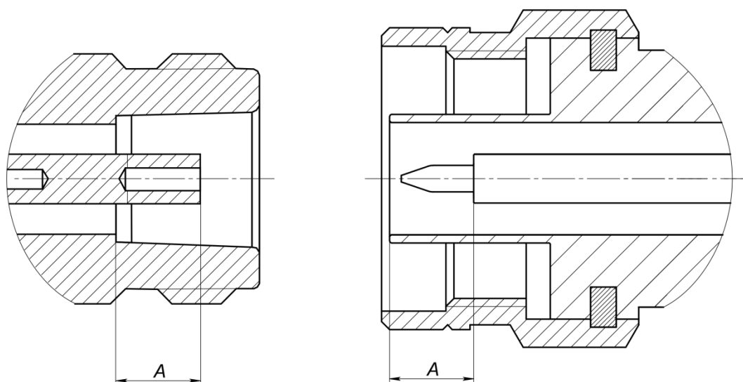
Рисунок 3.3 Соединители тип N и III (розетка и вилка)
