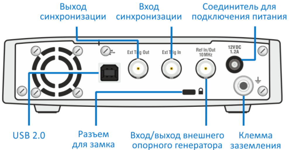
Рисунок 4.8 Задняя панель
