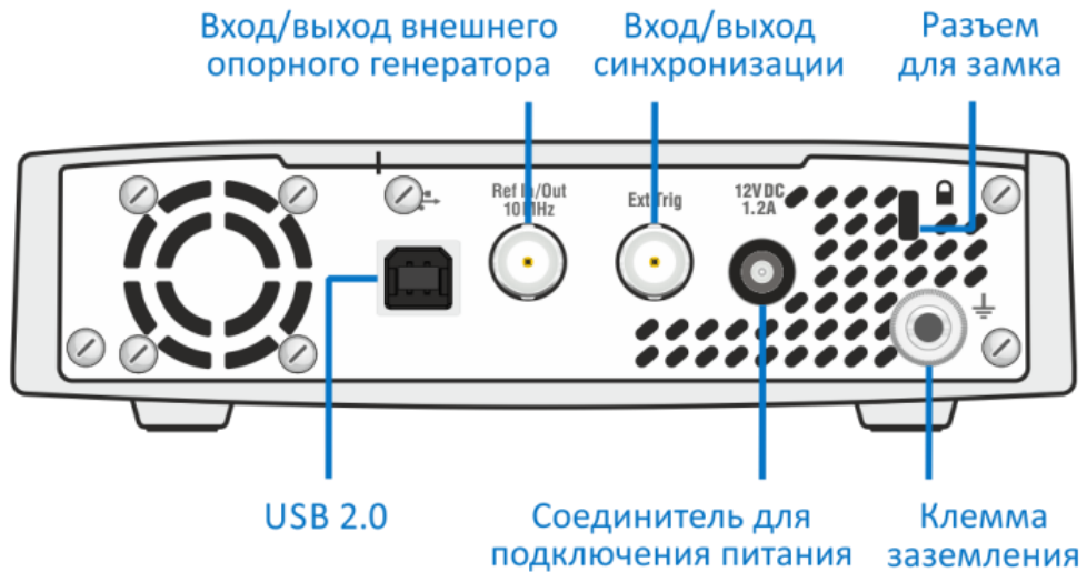
Рисунок 4.4 Задняя панель
