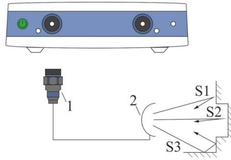
1 – Измерительный кабель 2 – Антенна
