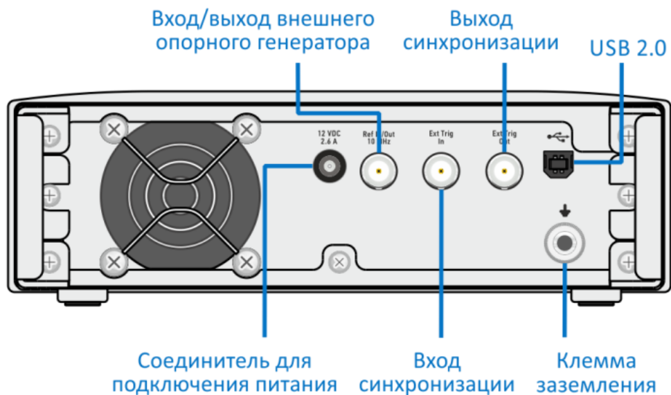
Рисунок 4.10 Задняя панель
