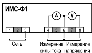
Рисунок 5.1 – Назначение клеммника
