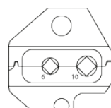
Die profile
