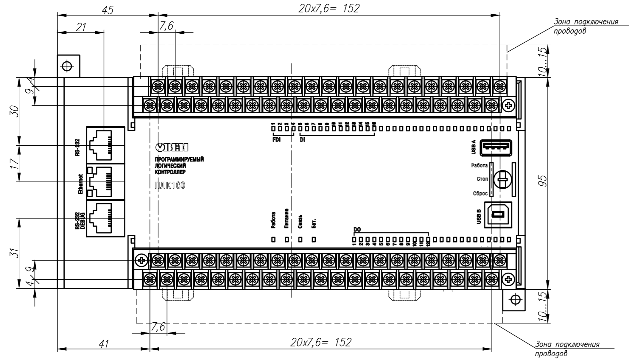
Расположение клемм, портов связи и зоны подключения Крышки клеммные условно не показаны
