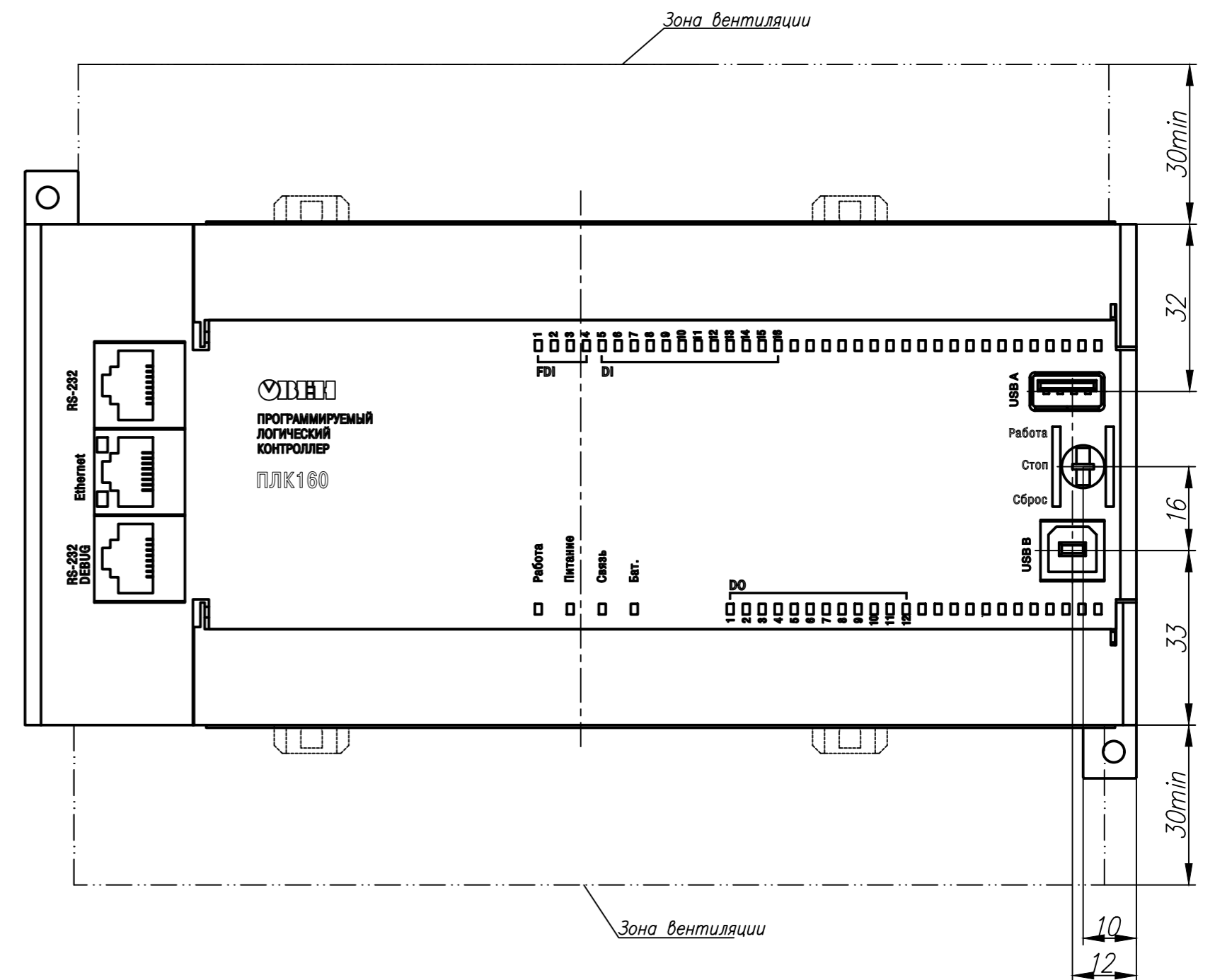
Расположение элементов индикации и управления и зоны вентиляции
