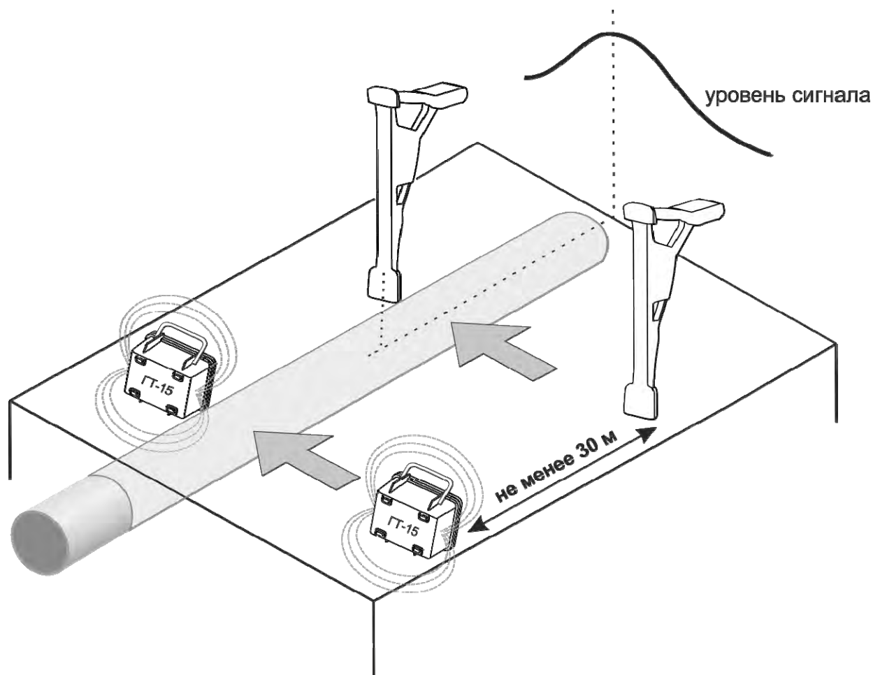
Рисунок 4.4.2.2 – Обследование участков местности с помощью ГТ-15
