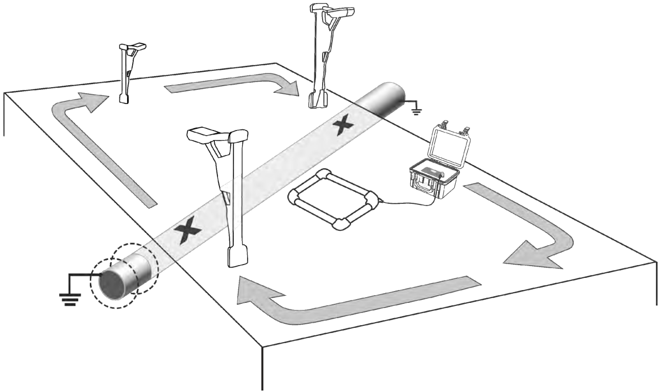
Рисунок 4.4.2.1 – Обследование участков местности с использованием рамки РП-02
