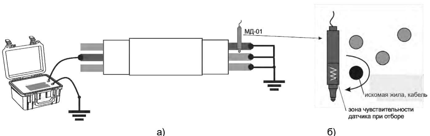
Рисунок 5.4.1 – Схема подключения при отборе жил кабеля
