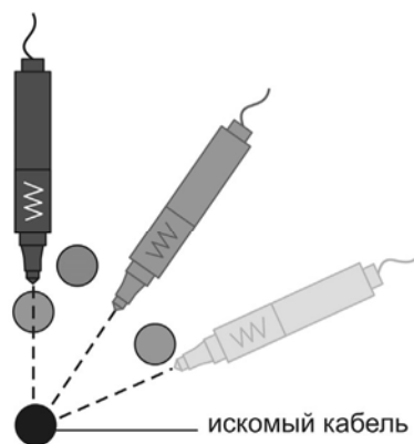
Рисунок 5.4.2 – Отбор жилы по минимуму сигнала
