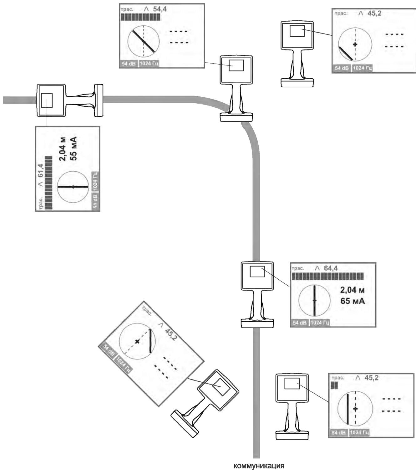
Рисунок 4.2.3 – Поиск с включенной функцией «КОМПАС»
