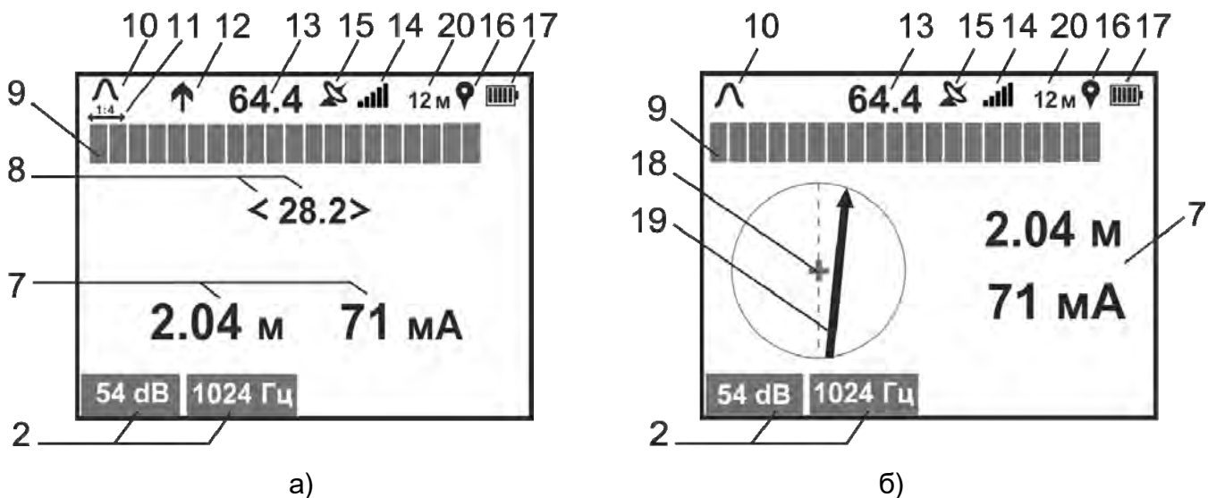
Рисунок 3.2 – Индикация приемника в режиме «ТРАССА»
