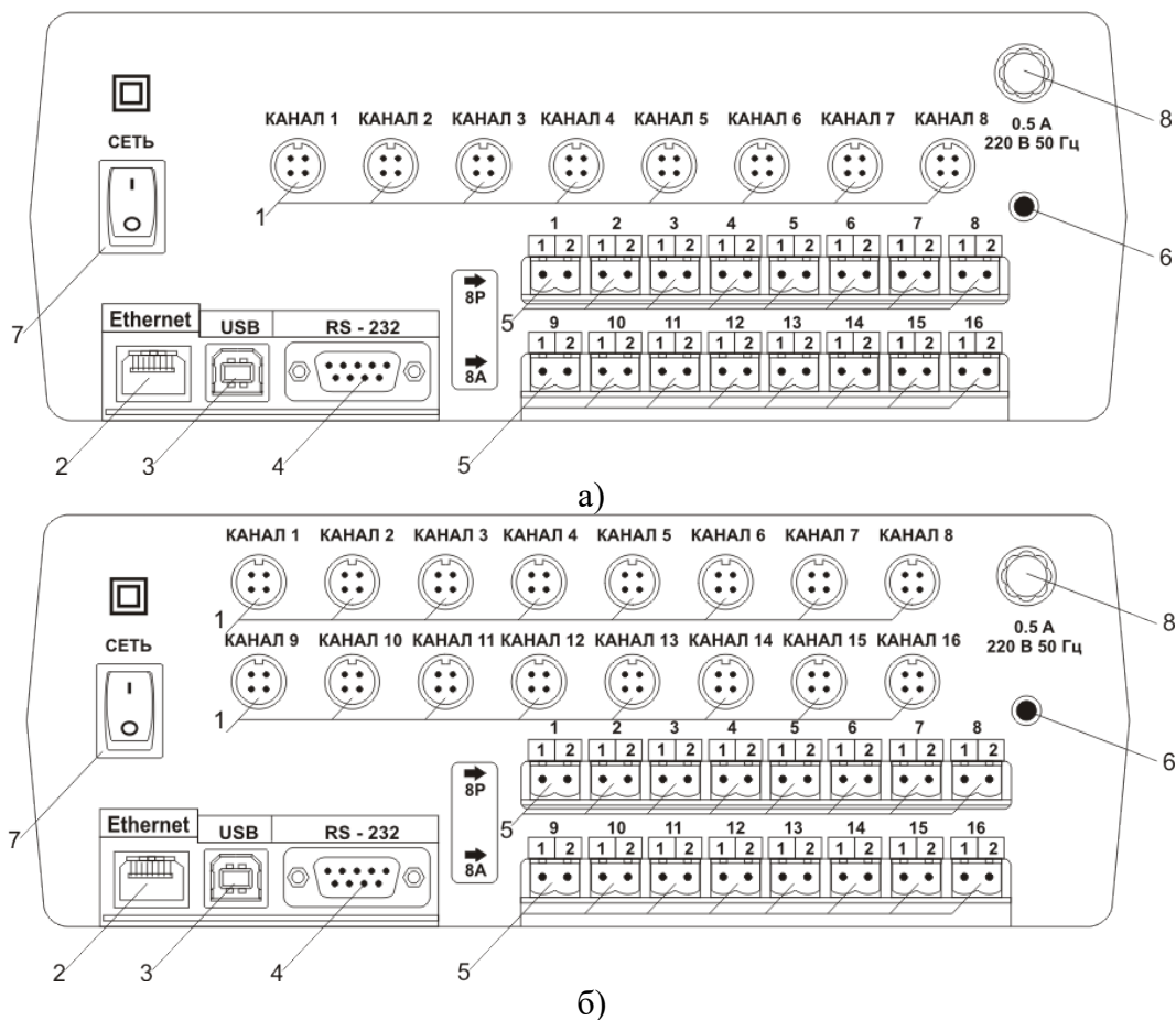
Рисунок 3.4 Вид задних панелей приборов ИВГ-1 /X-(B)-Т-8P-8A-E : а - четырехканального исполнения б - восьмиканального исполнения
