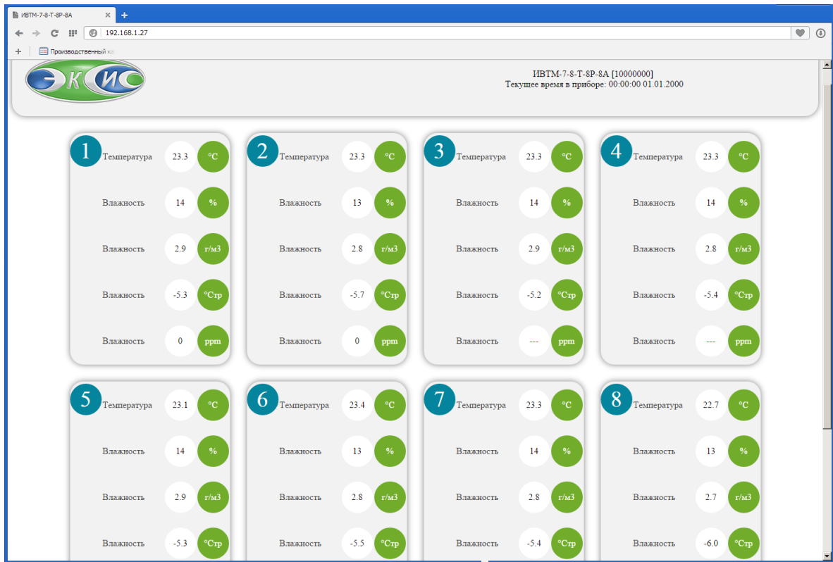
Рисунок 6.32 Web-интерфейс прибора ИВГ-1 /X-B-T-YP-ZA-E.
