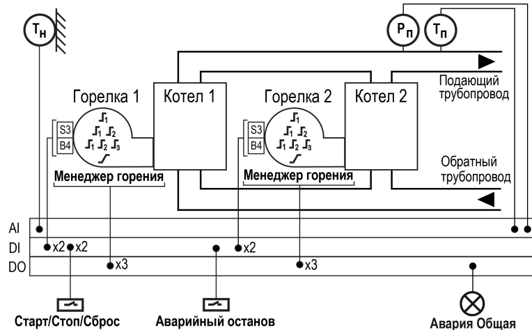
Рисунок 6.1 – Объект управления
