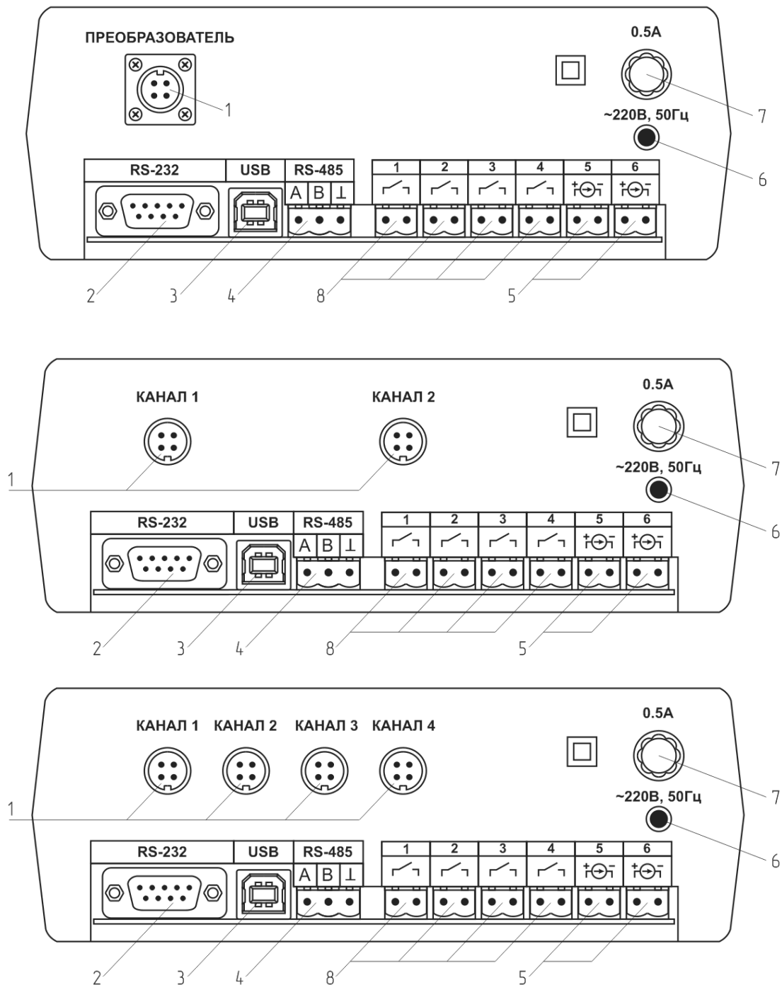
Рисунок 3.2 Задняя панель приборов ПКУ-4 /1-С-4Р-2А, ПКУ-4 /2-С-4Р-2А, ПКУ-4 /-С-4Р-2А (сверху вниз)
