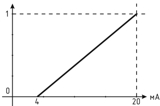
Рисунок 6.26 Пример настройки линейного выхода
