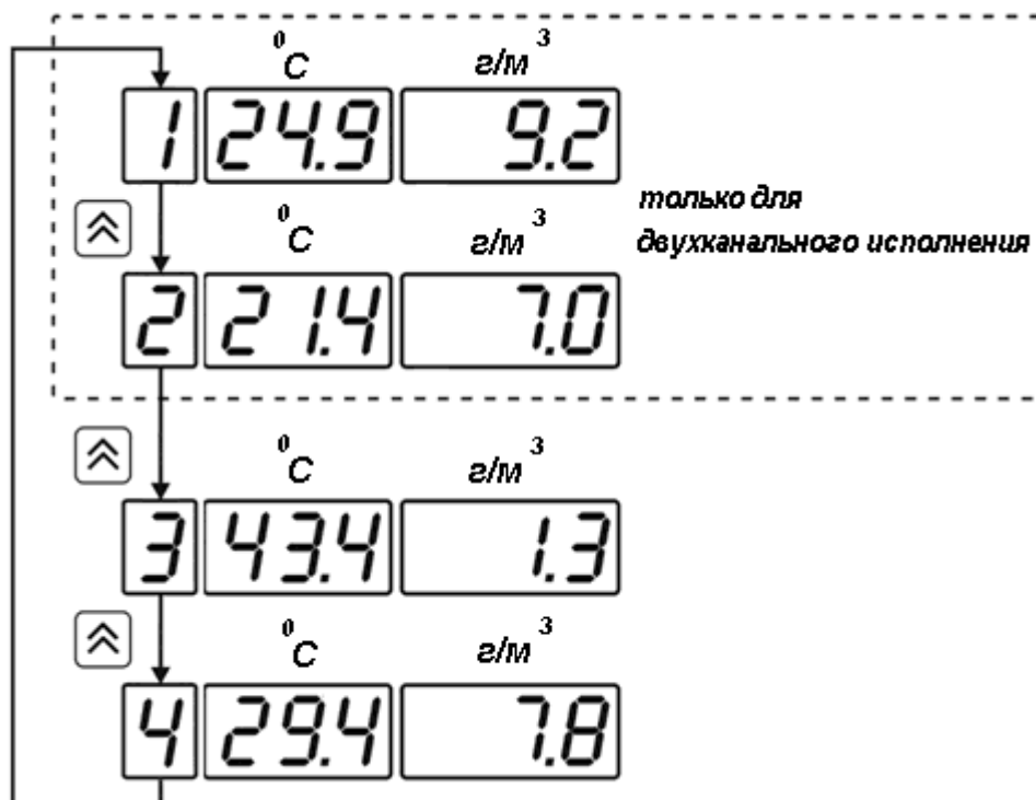
Рисунок 6.2 Выбор канала индикации измерения
