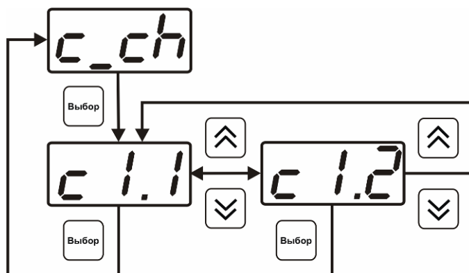
Рисунок 6.16 Настройка входного параметра канала управления (реле)
