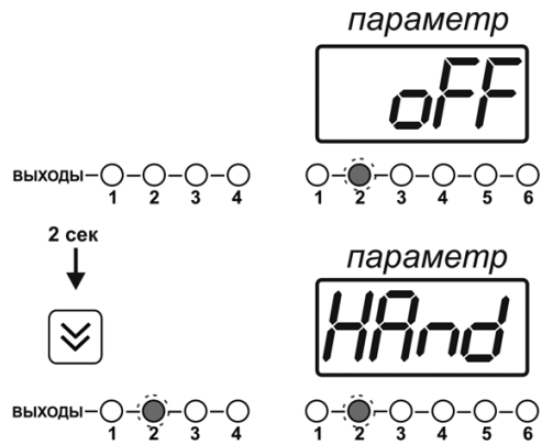
Рисунок 6.3 Ручное включение исполнительного устройства второго канала управления
