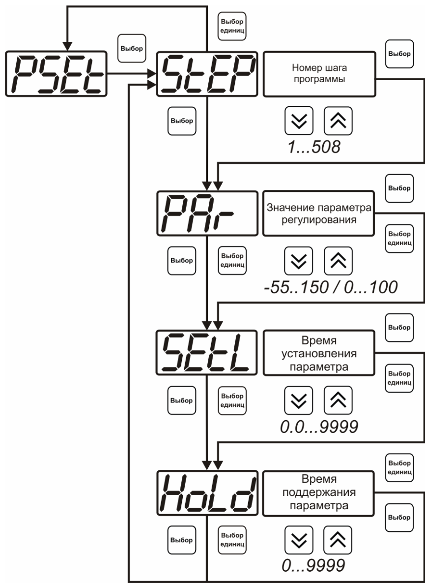
Рисунок 6.34 Меню настройки программы
