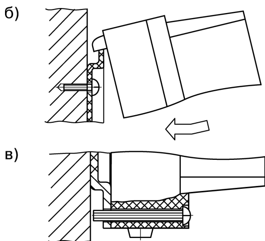
Рисунок 8.1 – Установка прибора настенного крепления
