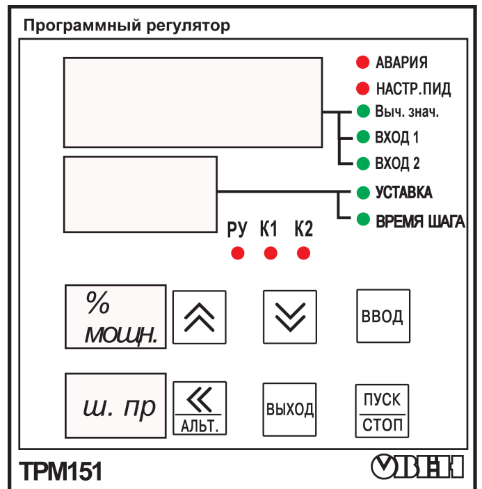
Рисунок 6.2 – Вариант 1 индикации прибора
