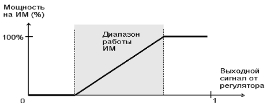
Рисунок 3.15 - Работа ИМ (тип «Нагреватель») в заданном диапазоне
