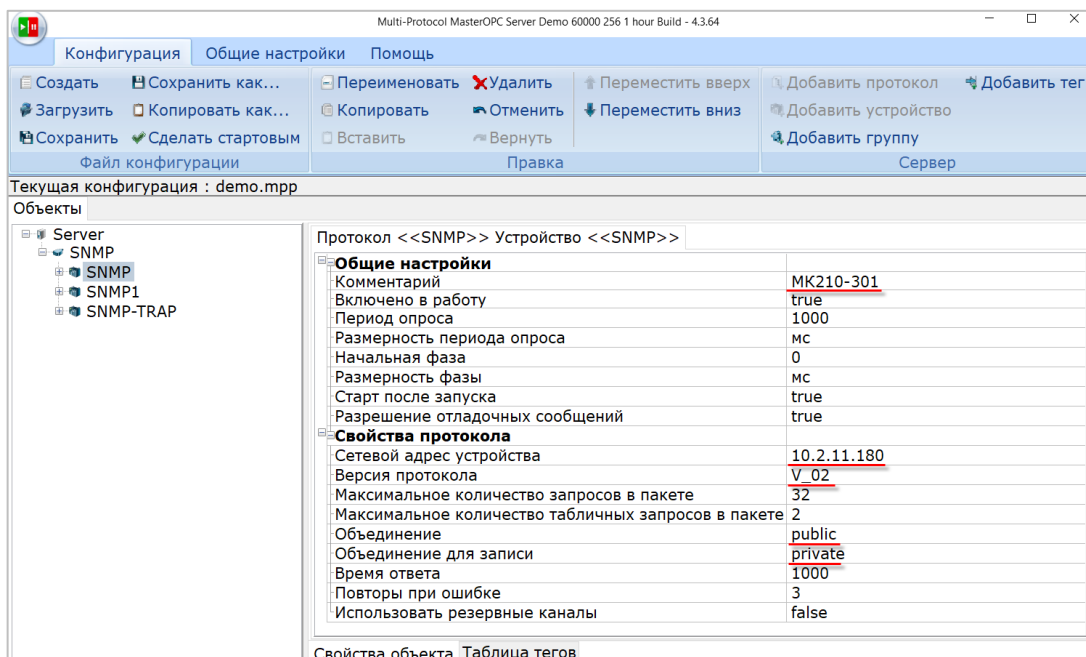
Рис. 6.6. Настройки модуля MK210-301 в OPC-сервере
