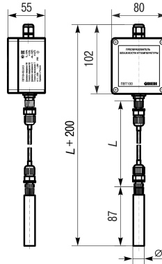
Рисунок 3 – Габаритные и установочные размеры исполнения H5 со стандартным кабелем
