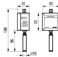
Рисунок 2 – Габаритные и установочные размеры исполнения H4
