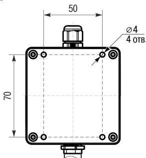
Рисунок 5 – Монтажные отверстия
