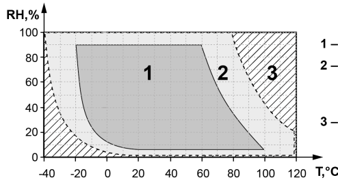
Рисунок 6 – Рекомендуемые условия эксплуатации
