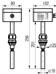
Рисунок 1 – Габаритные и установочные размеры исполнения K1
