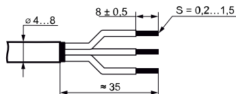
Рисунок 7 – Подготовка провода
