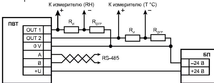
Рисунок 8 – Схема подключения
