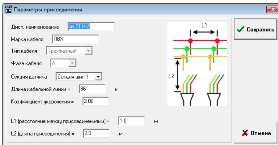
Рисунок 29 Параметры кабельной линии
