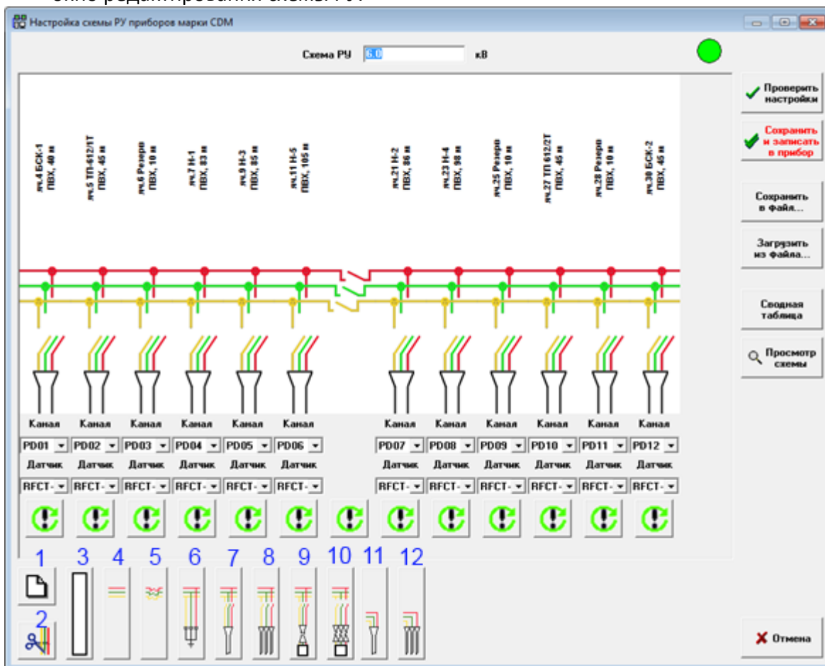
Рисунок 28 Создание или редактирование схемы КРУ
